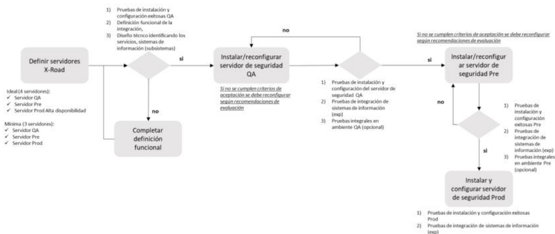
Figura 1 – Diagrama de proceso de implementación de X-ROAD
